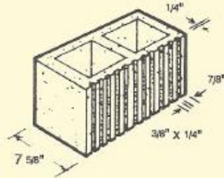
8 x 8 x 16 Lido
